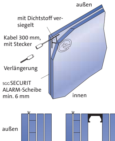
SGG SECURIT ALARM mit Randanschluss ASR-Typ A VdS-Anerkennungs-Nr. G 180030.
